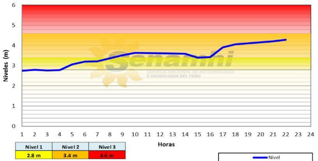
NIVELES HORARIOS DEL RÍO HUALLAGA ESTACIÓN TINGO MARÍA
