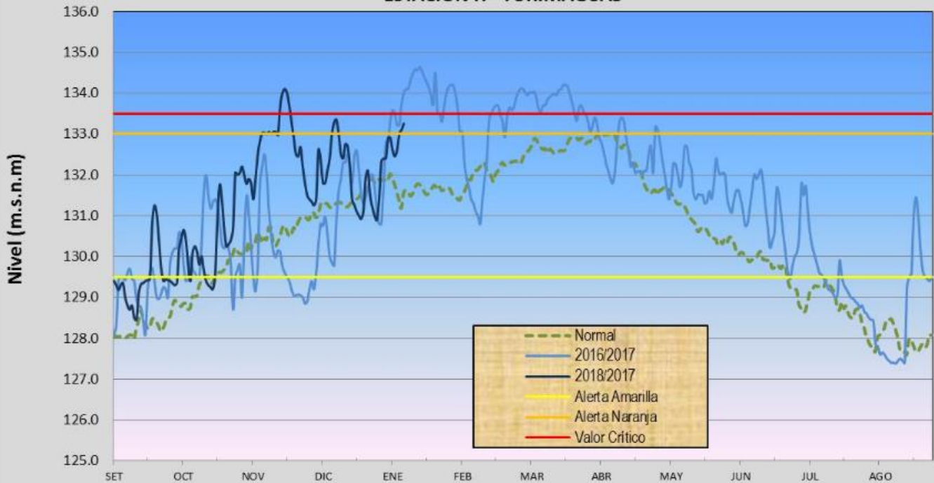
HIDROGRAMA DE NIVELES DE AGUA DEL RÍO HUALLAGA ESTACIÓN H - YURIMAGUAS
